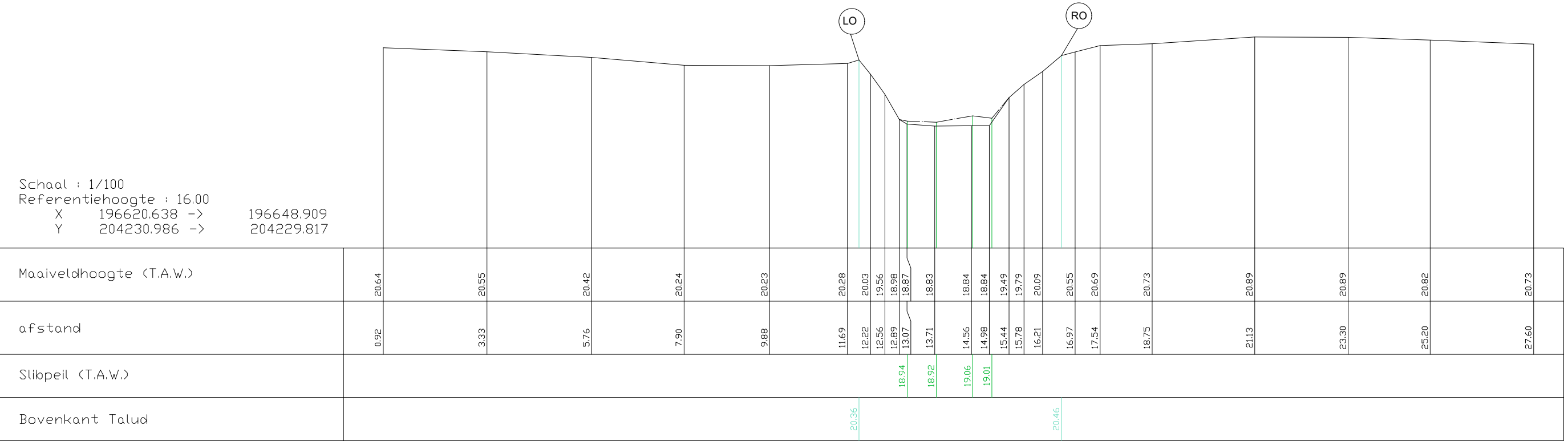
Pad ref: Dwarsprofiel 1
