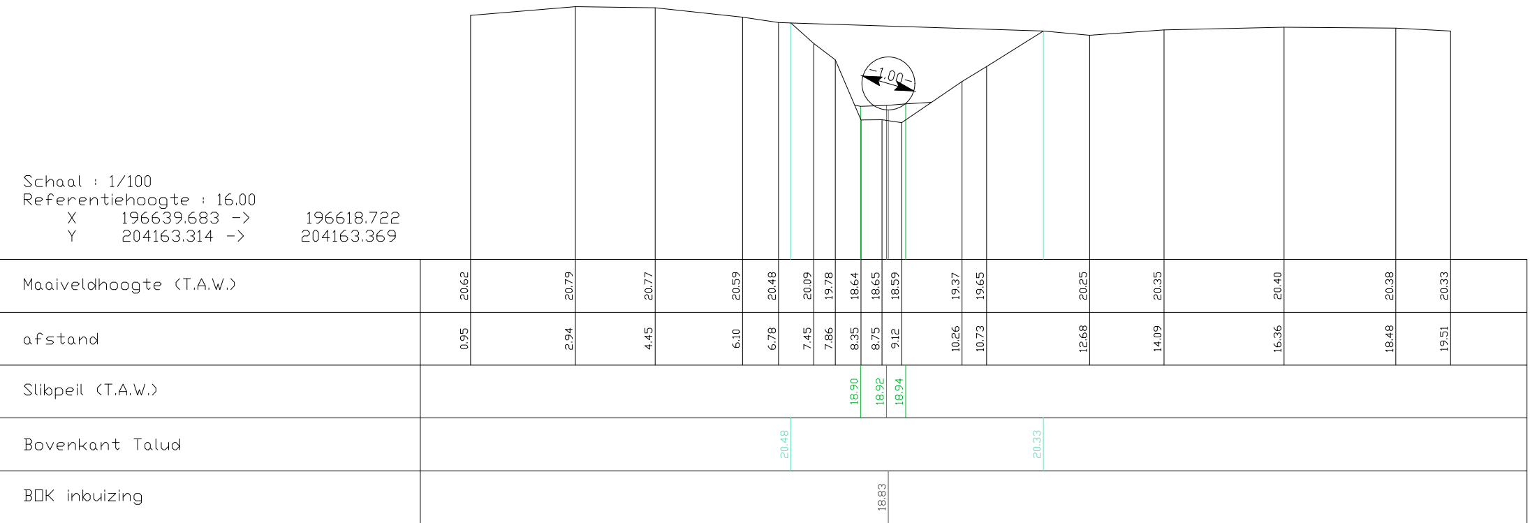
Pad ref: Dwarsprofiel 3
