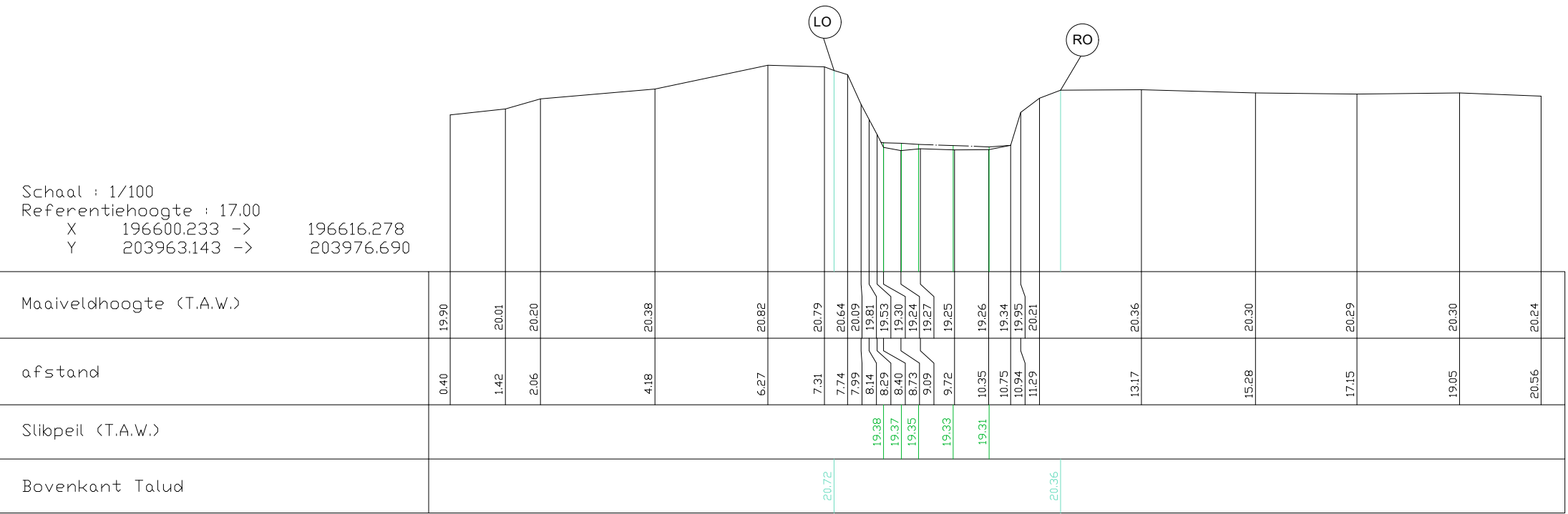
Pad ref: Dwarsprofiel 9
