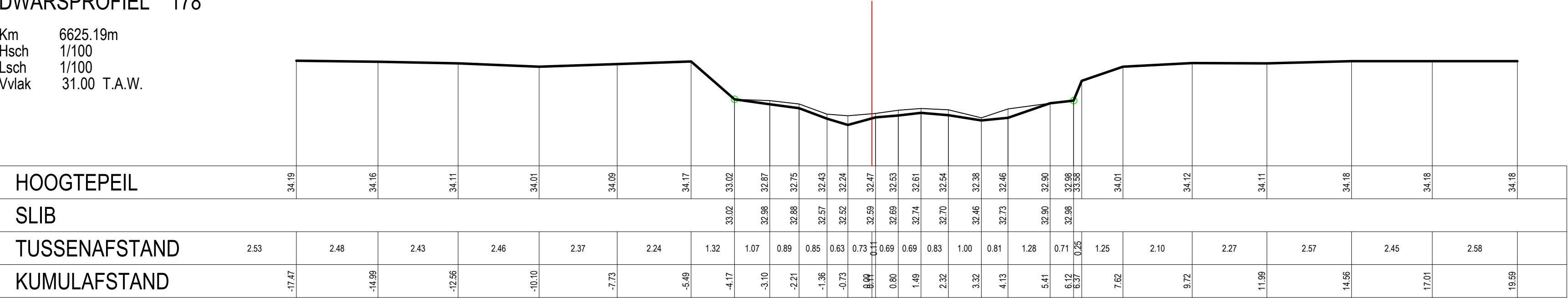
DWARSPROFIEL 178
