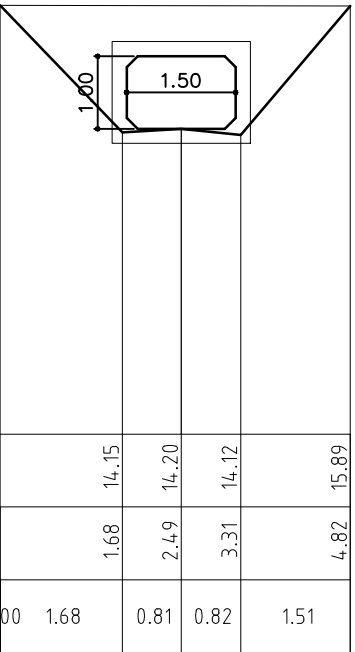
DWARSPROFIEL 13
