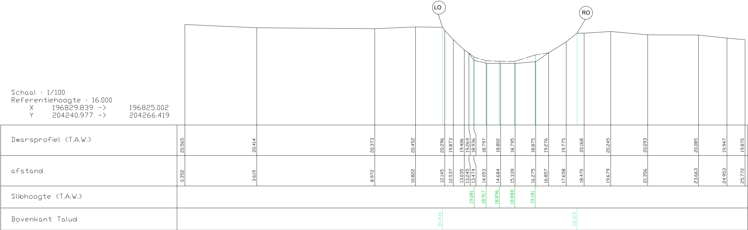
Pad ref: Dwarsprofiel 41
