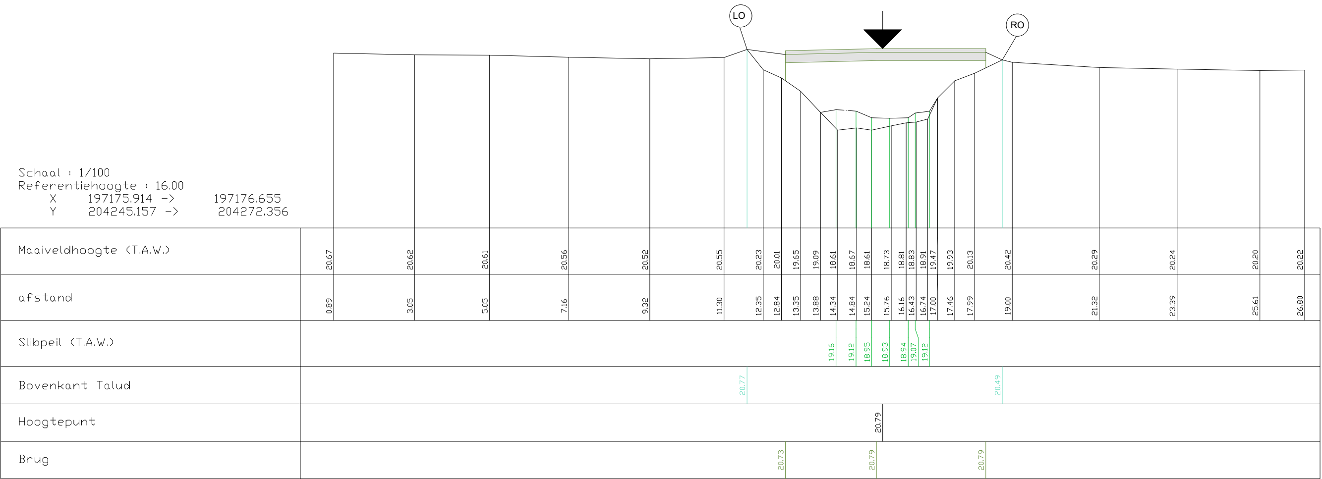
Pad ref: Dwarsprofiel 56
