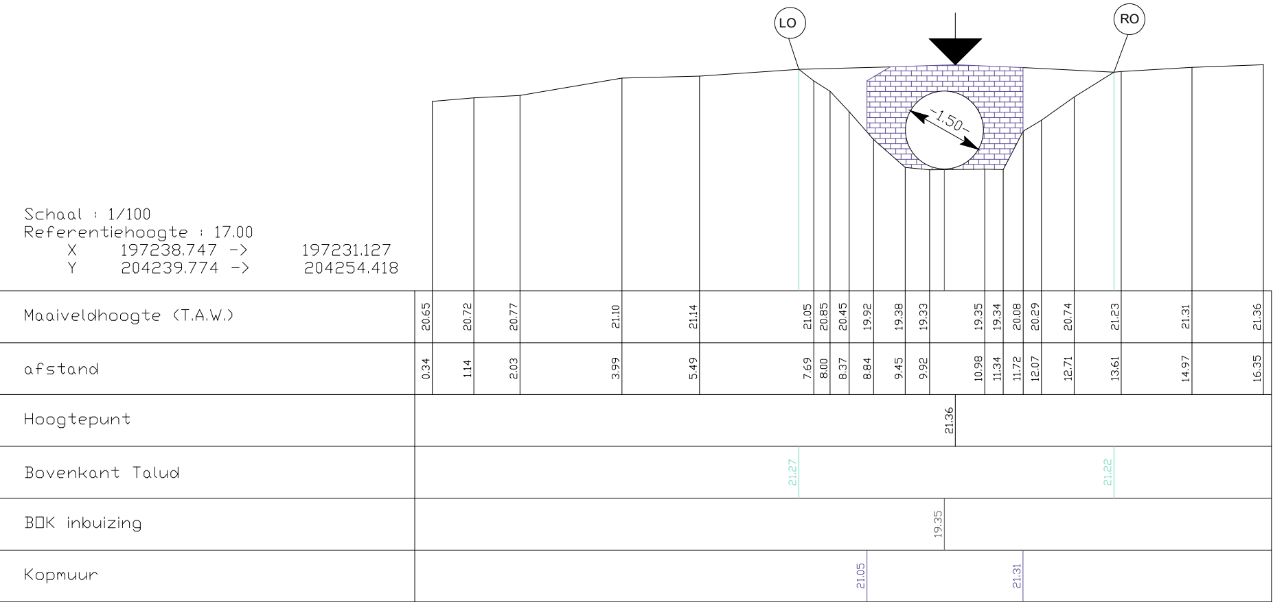
Pad ref: Dwarsprofiel 59
