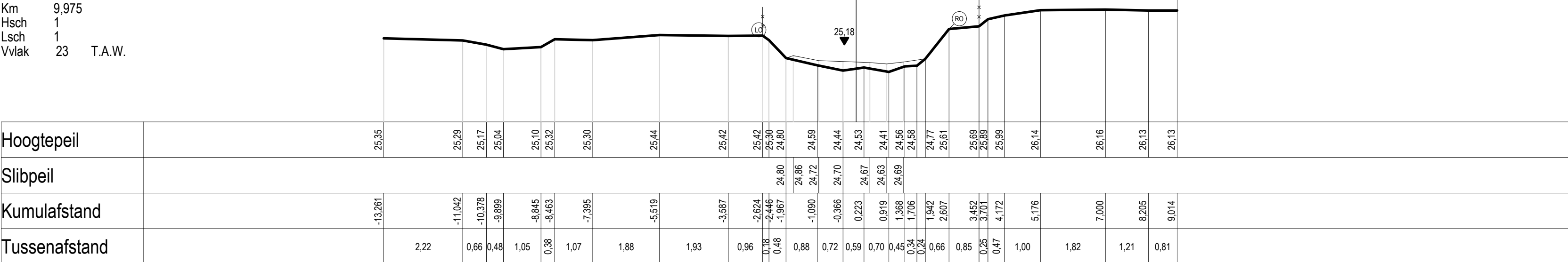
DWARSPROFIEL 252
