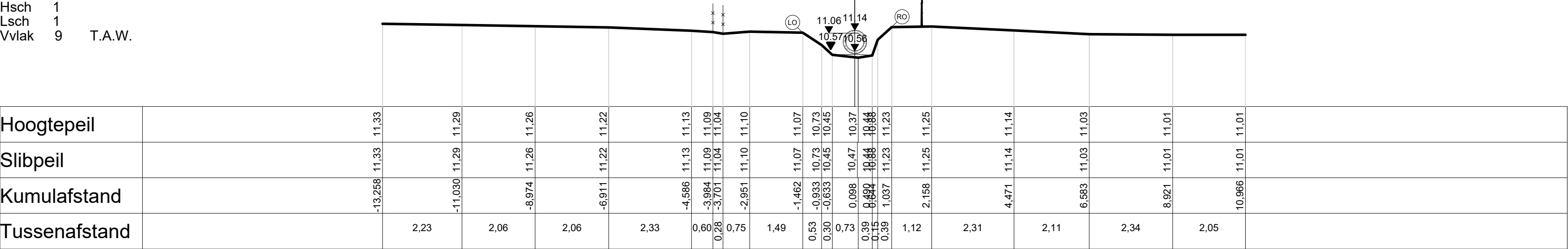
DWARSPROFIEL 100
