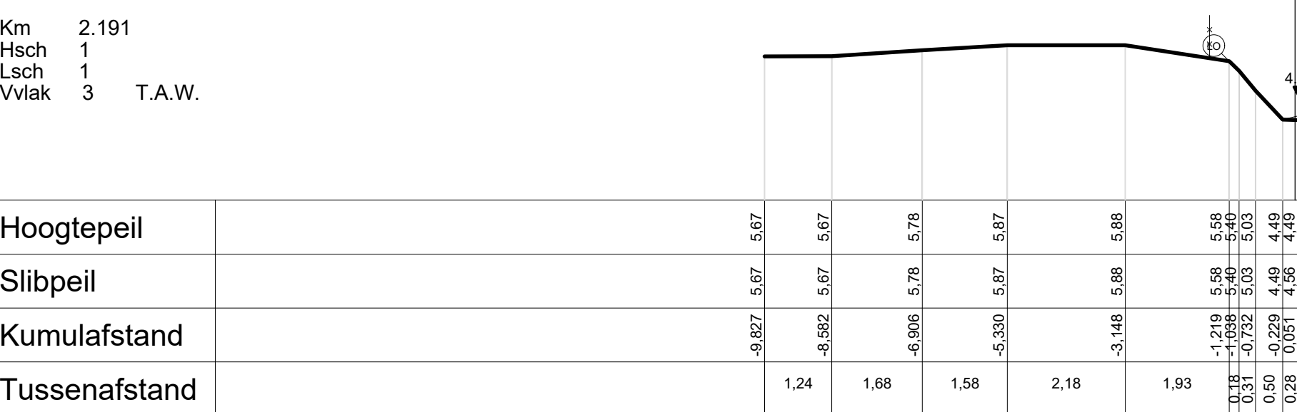
DWARSPROFIEL 61
