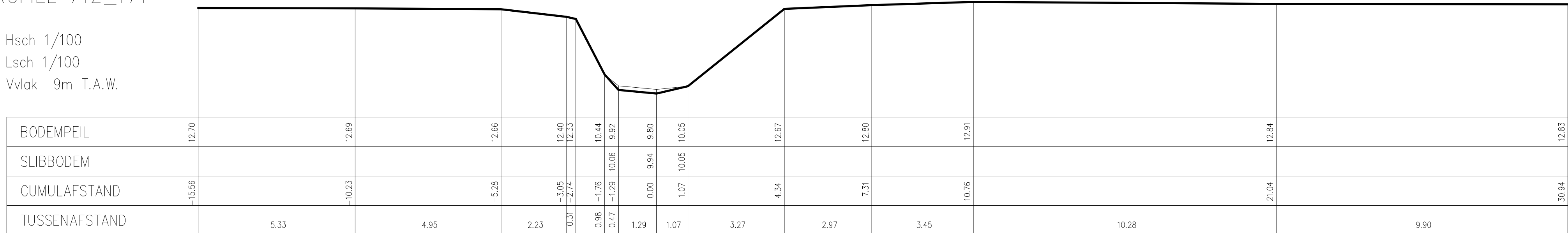
DWARSPROFIEL 712_171
