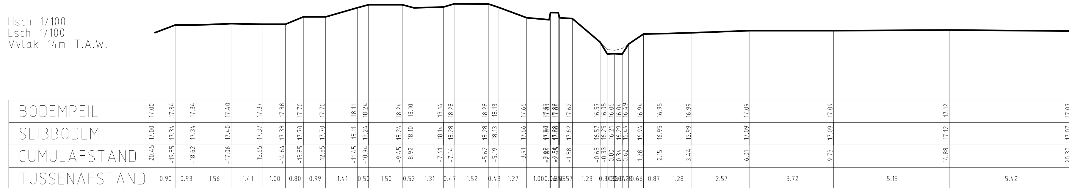
DWARSPROFIEL 102
