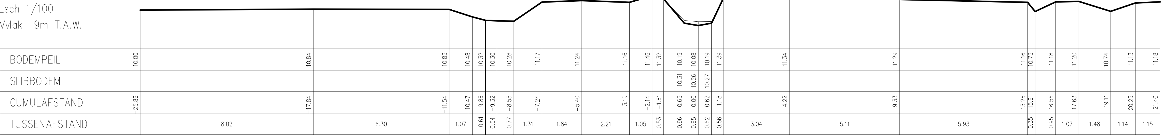
DWARSPROFIEL 7.12.1_22
