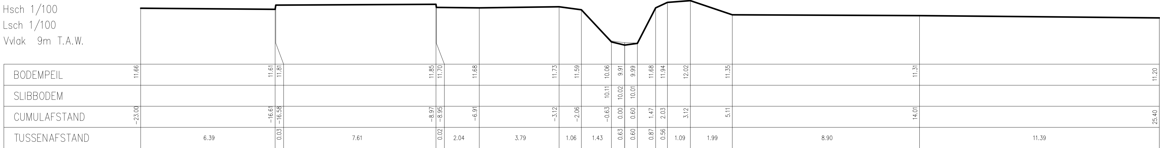
DWARSPROFIEL 7.12.1_2
