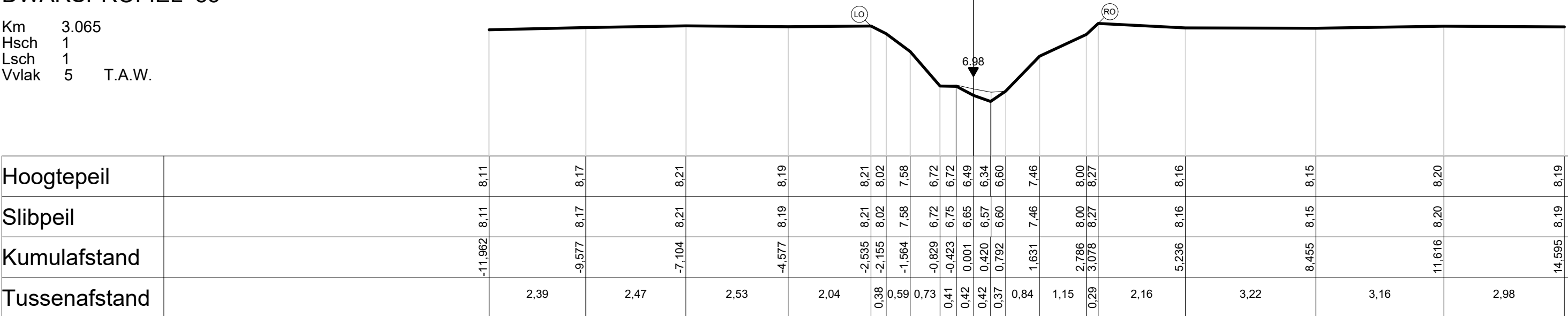
DWARSPROFIEL 85
