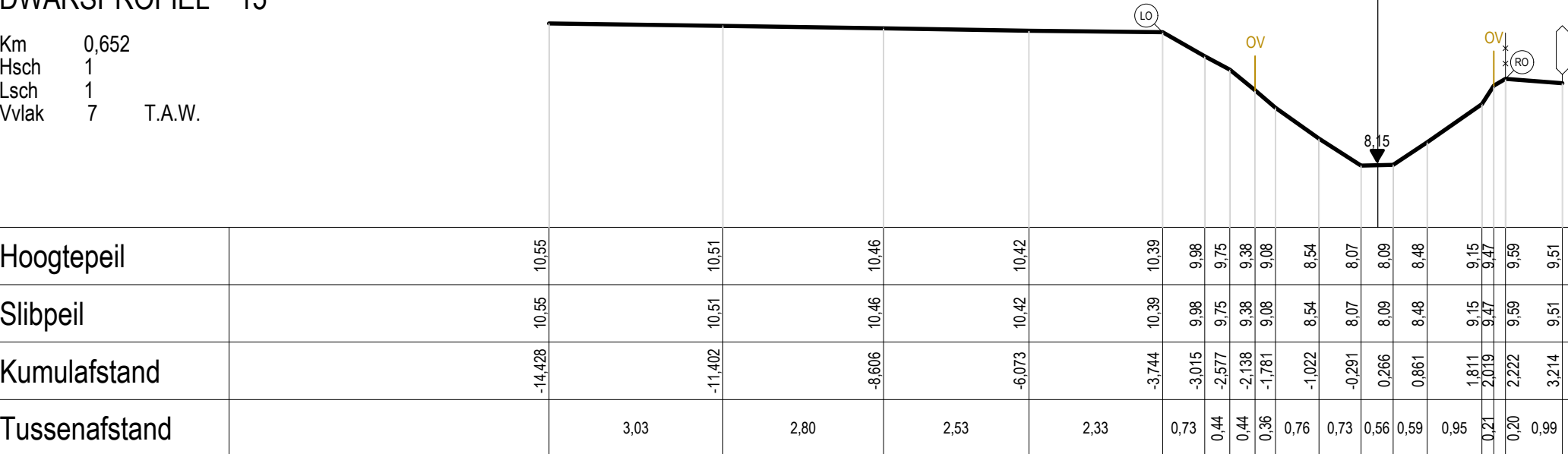
DWARSPROFIEL 15
