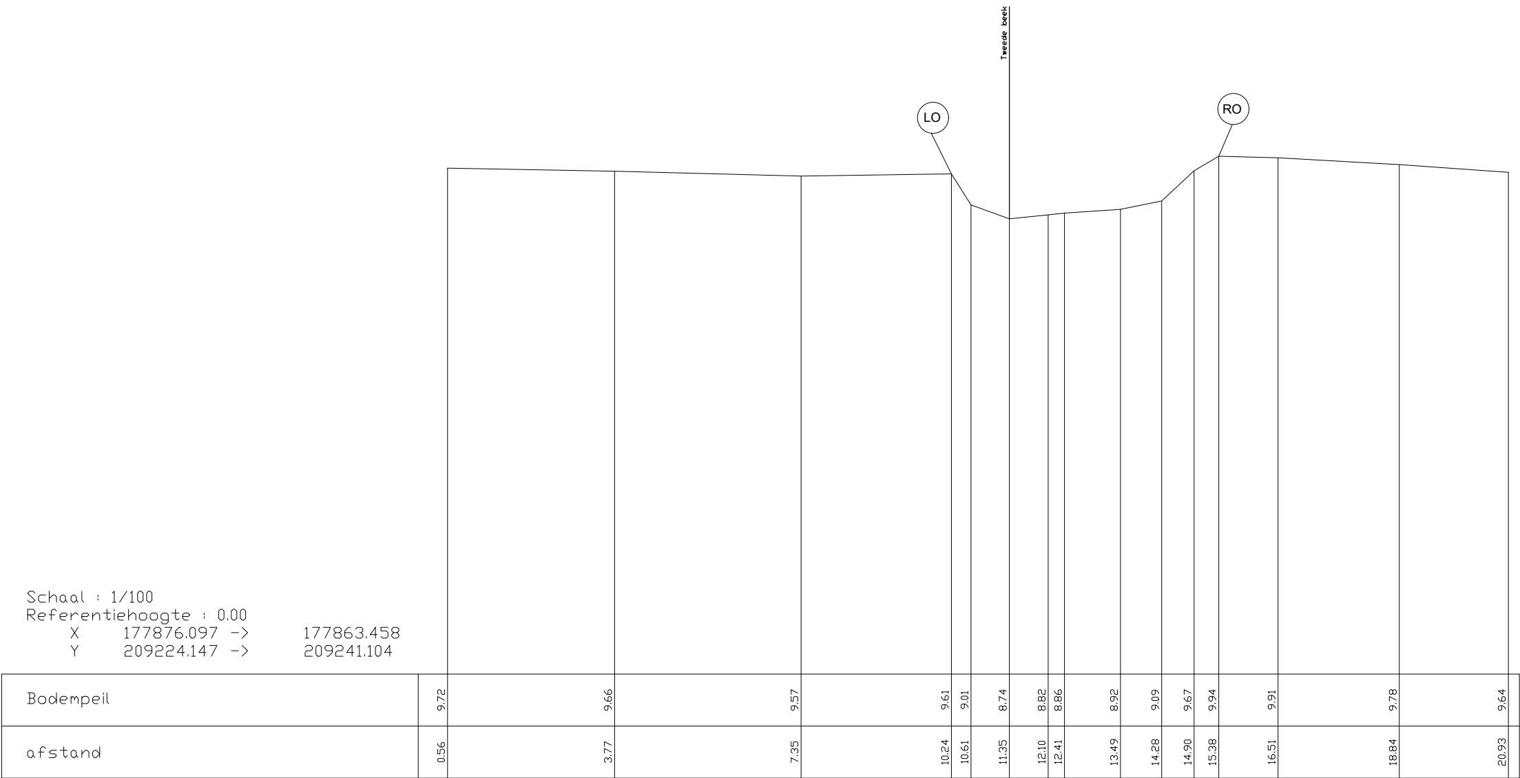
Pad ref: Tweede Beek Dwarsprofiel 1
