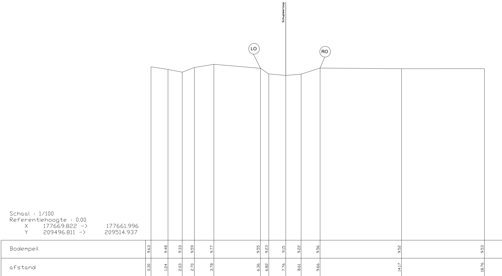
Pad ref: Schupleerloop Dwarsprofiel 2
