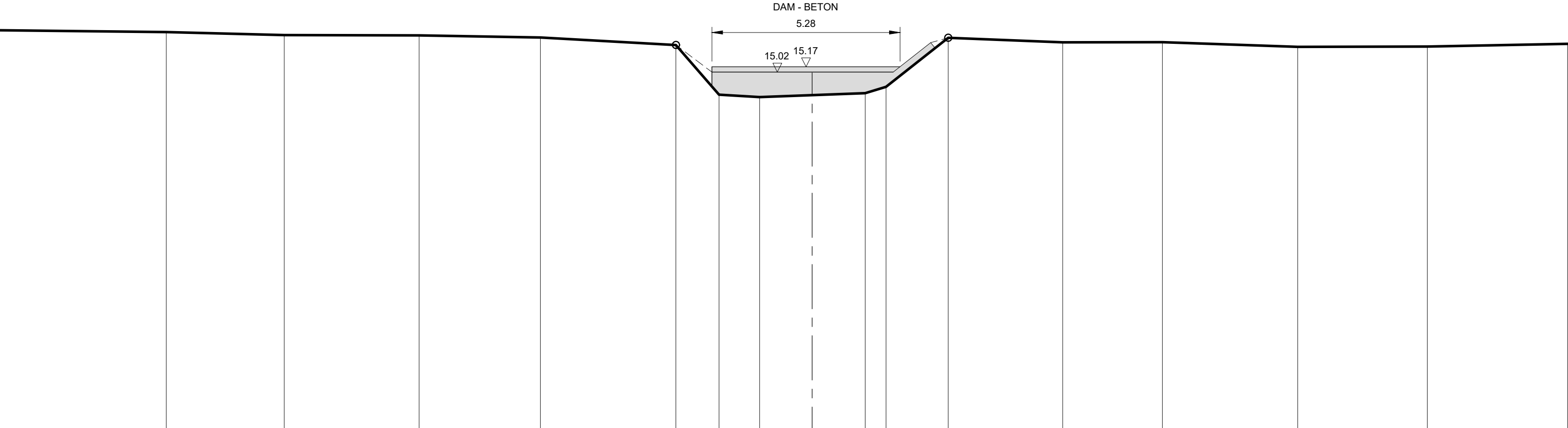
DWARSPROFIEL 131
