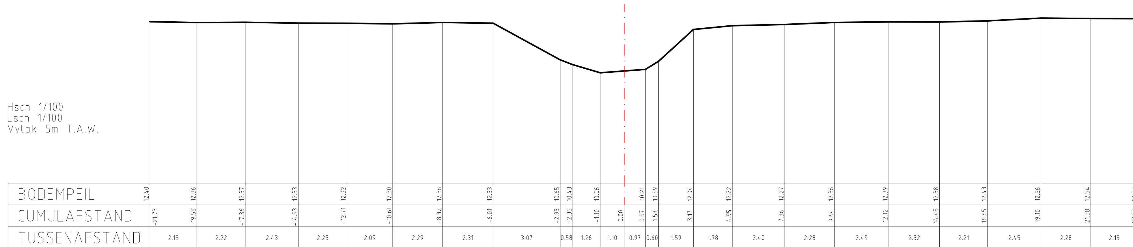
DWARSPROFIEL 2
