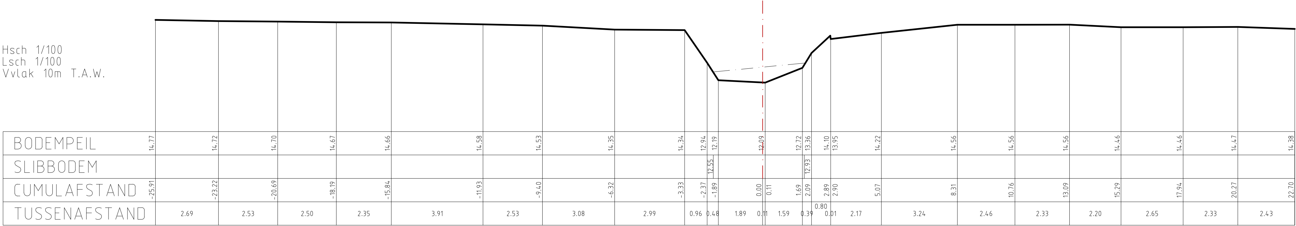
DWARSPROFIEL 33
