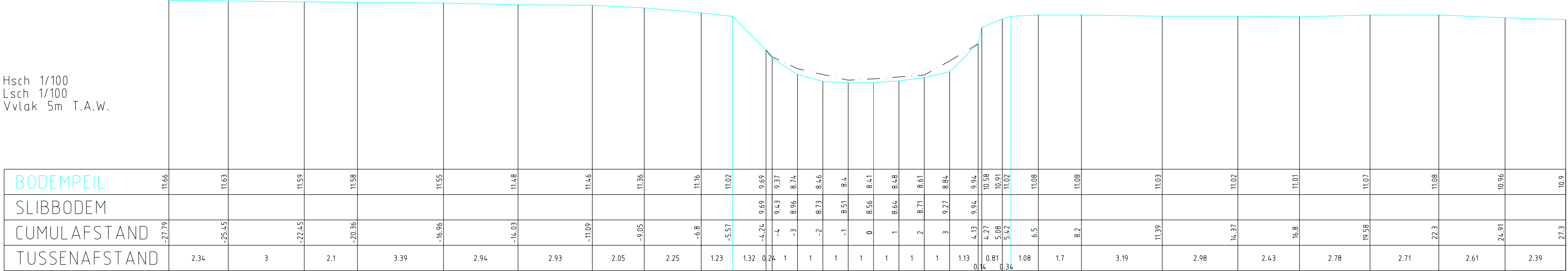
DWARSPROFIEL 126 (na brug (KW 541/21.000-40))
