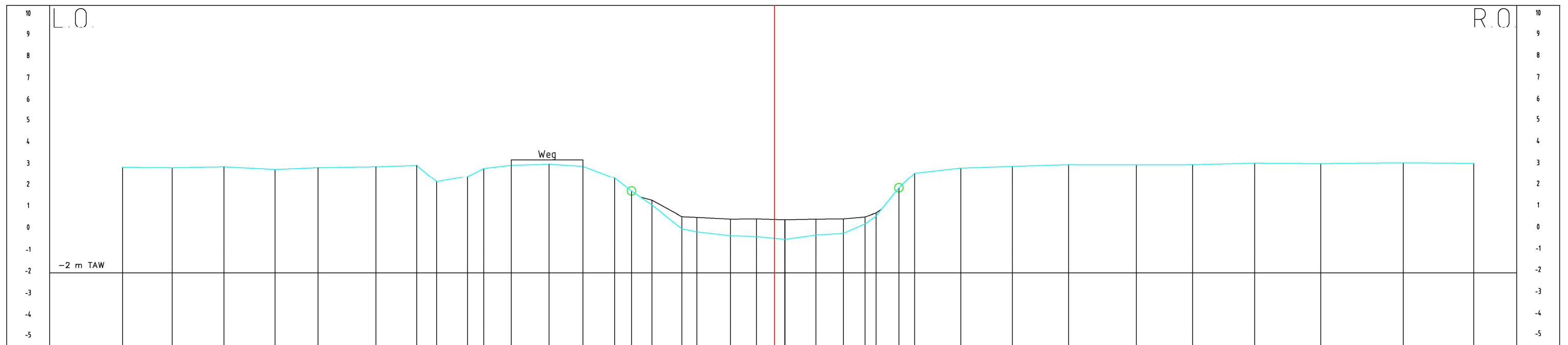
Profiel 103
