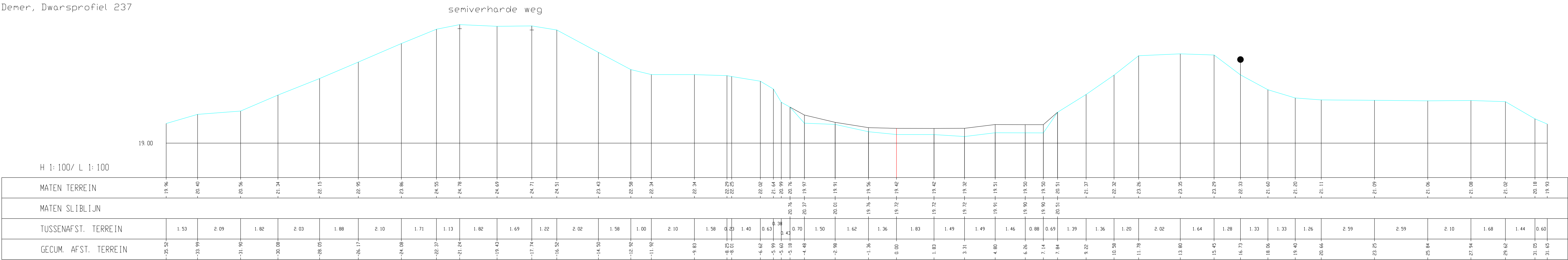
Demer, Dwarsprofiel 237
