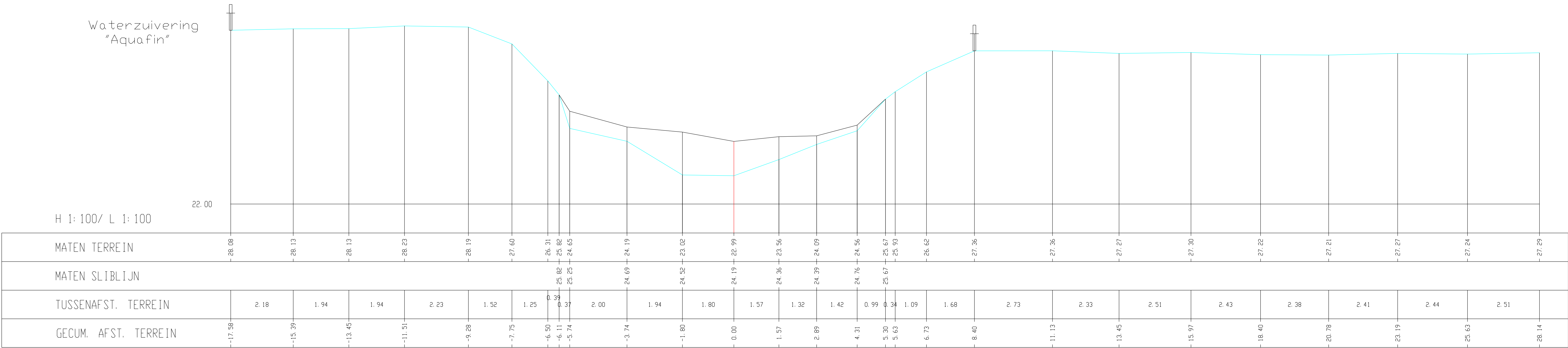
Demer, Dwarsprofiel 463
