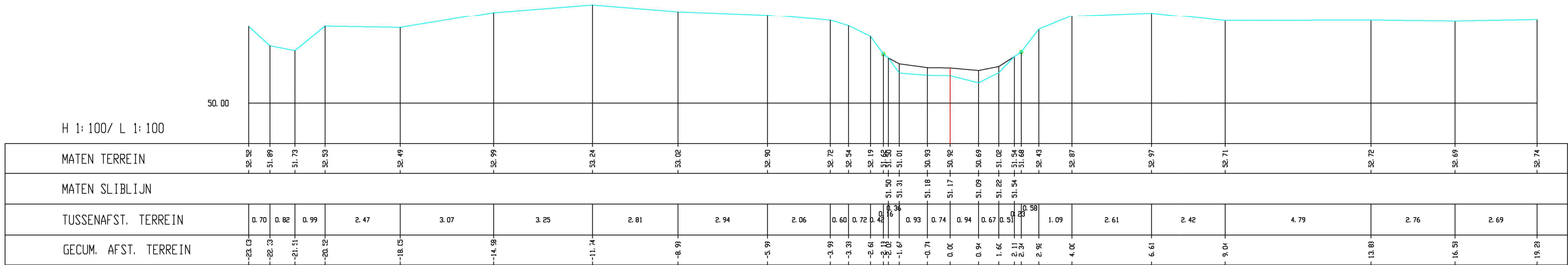
Dommel, Dwarsprofiel 435
