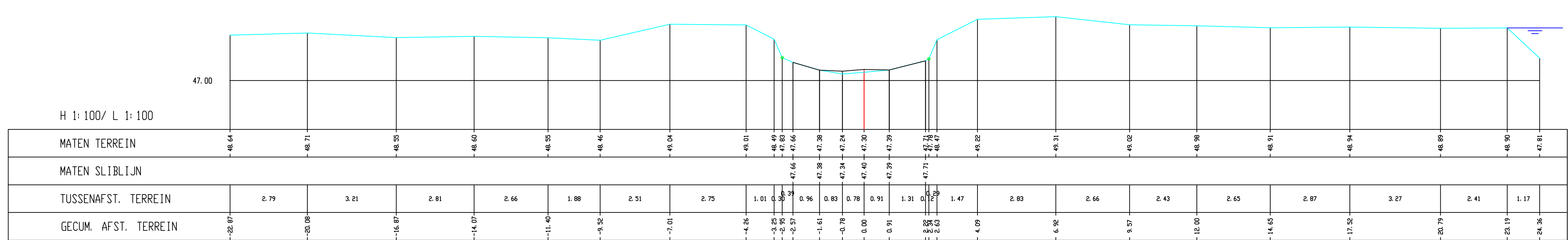
Donnel, Dwarsprofiel 367
