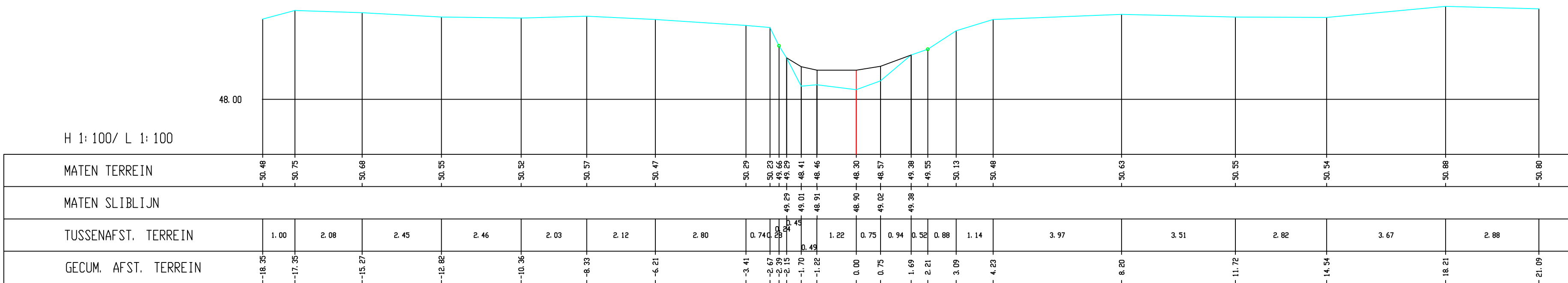
Dommel, Dwarsprofiel 403
