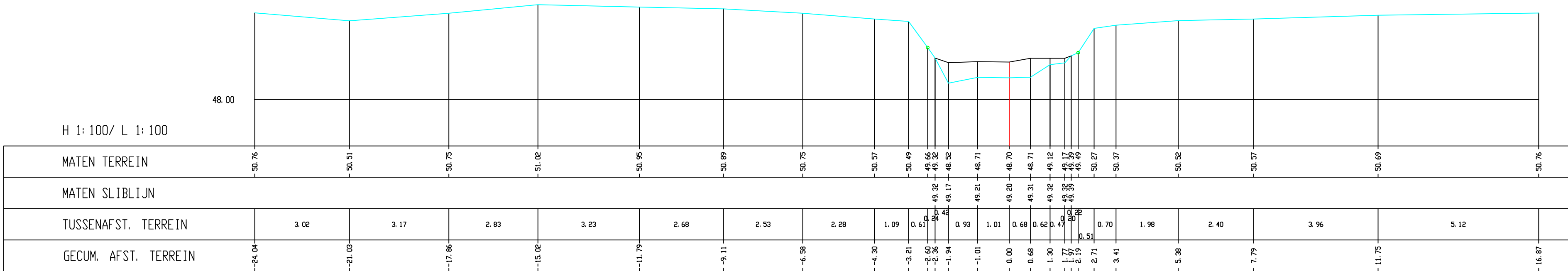
Dommel, Dwarsprofiel 404
