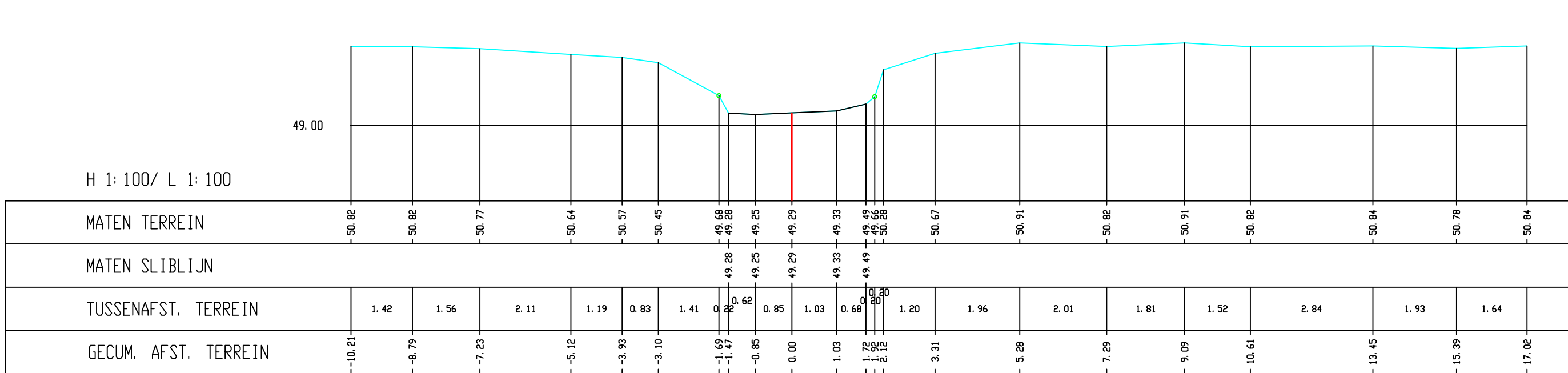
Dommel, Dwarsprofiel 407a
