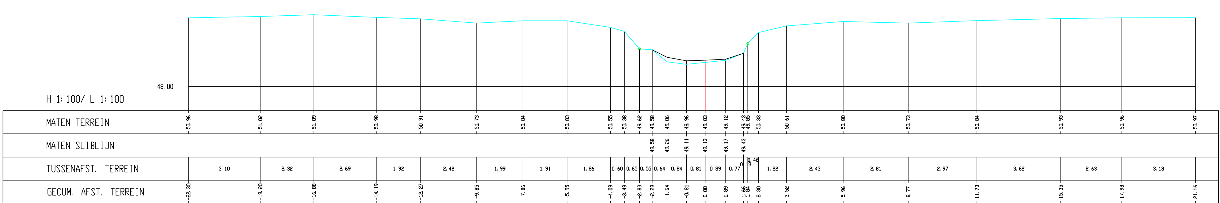
Dommel, Dwarsprofiel 407
