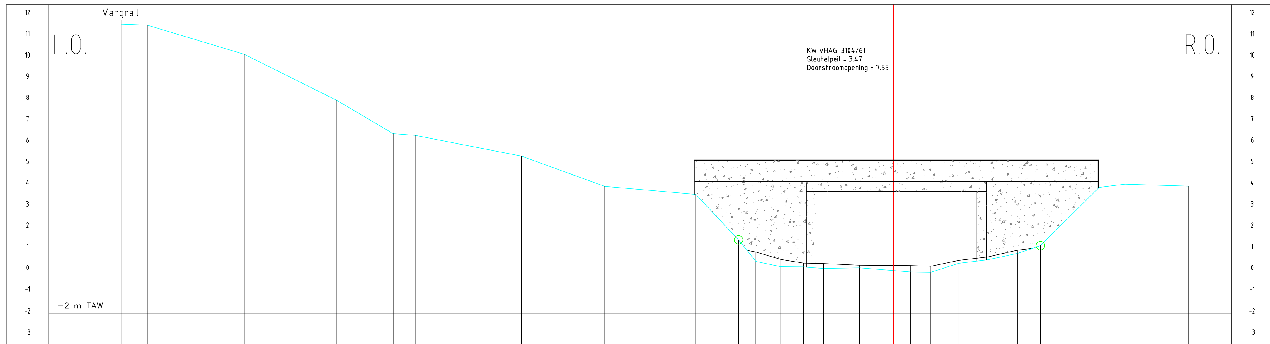
Profiel 104'
