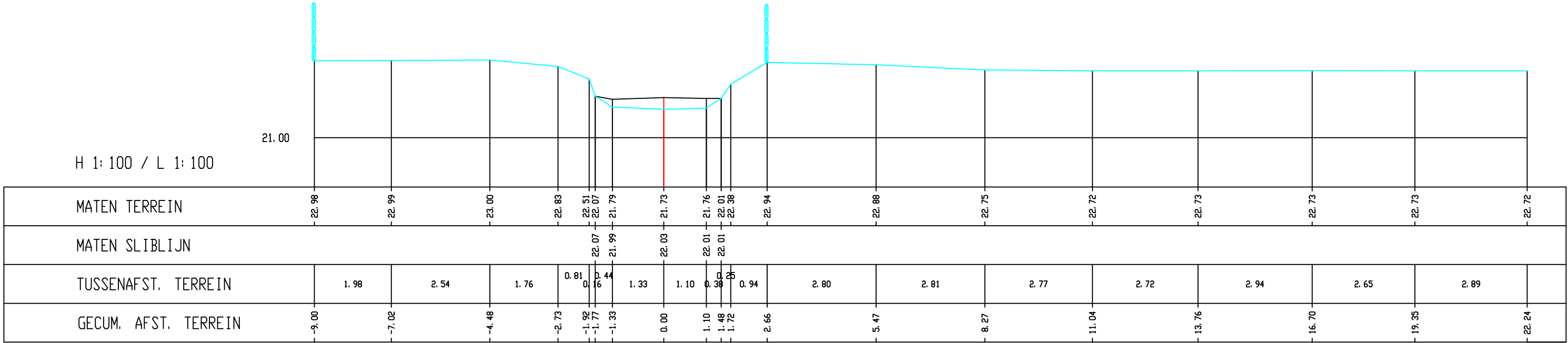
Winterbeek, Dwarsprofiel K25
