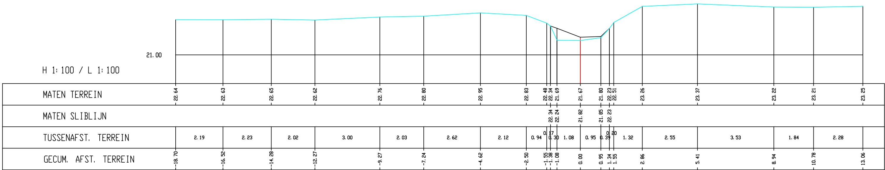
Winterbeek, Dwarsprofiel K27
