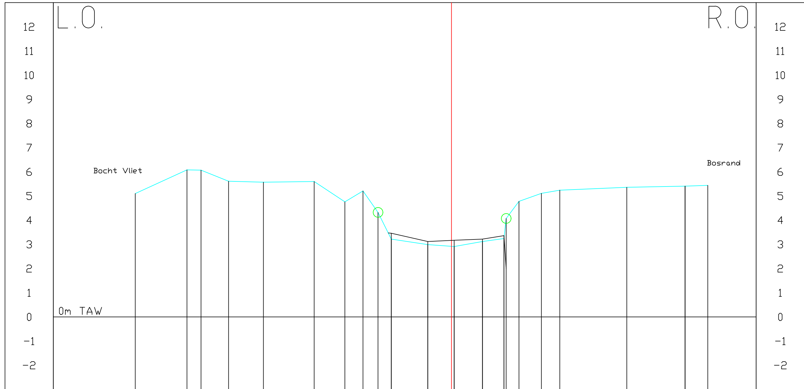
Profil 58
