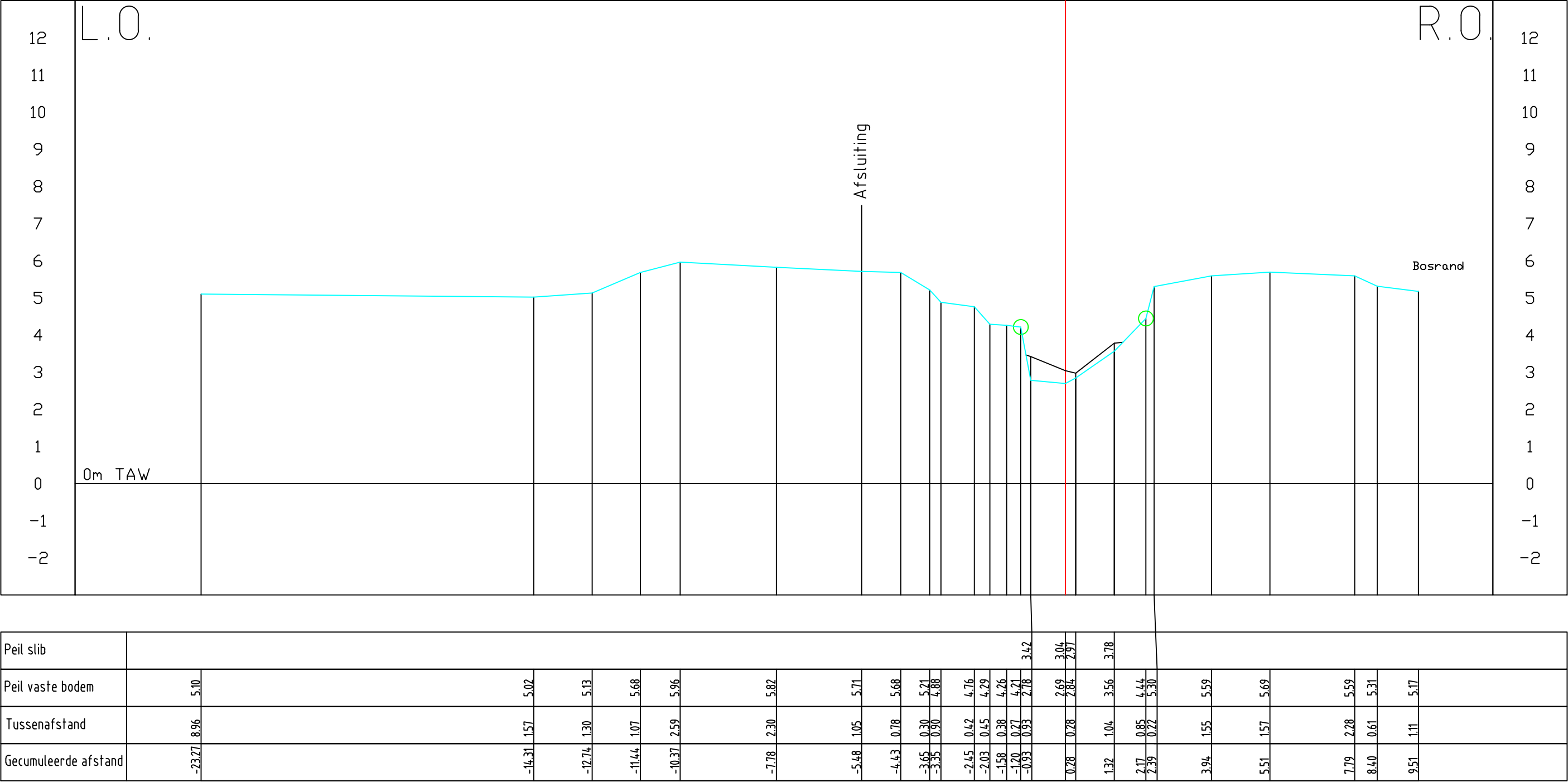
Profiel 63
