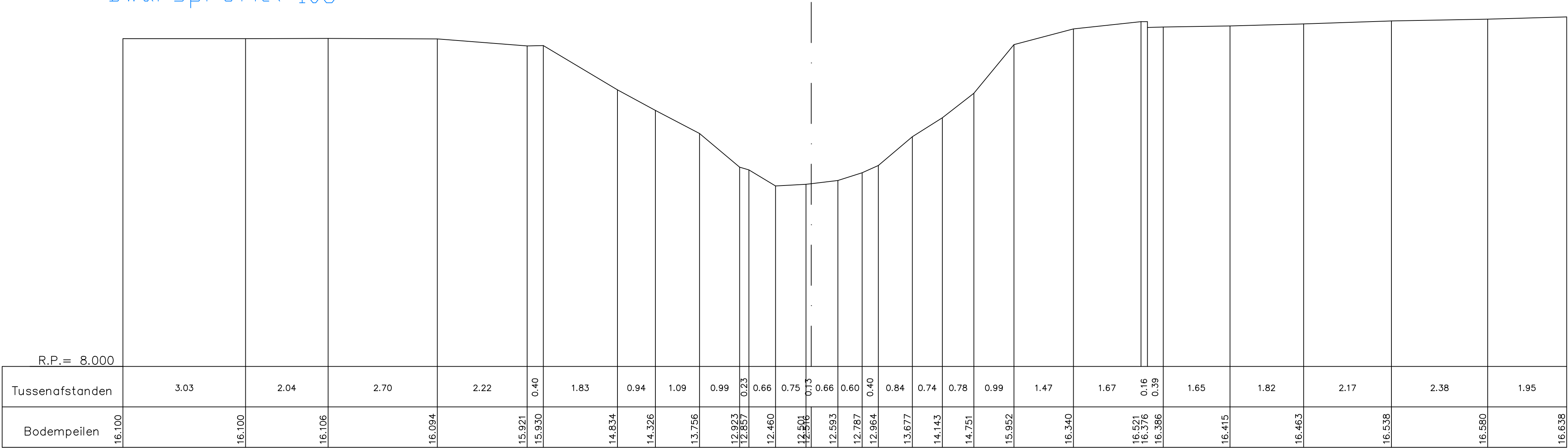
Dwarsprofiel 105
