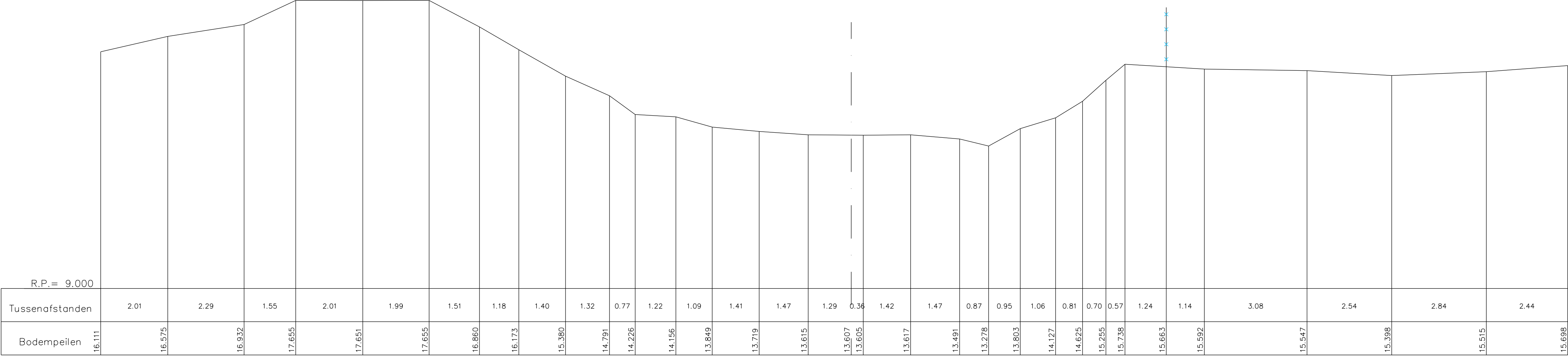
Dwarsprofiel 164
