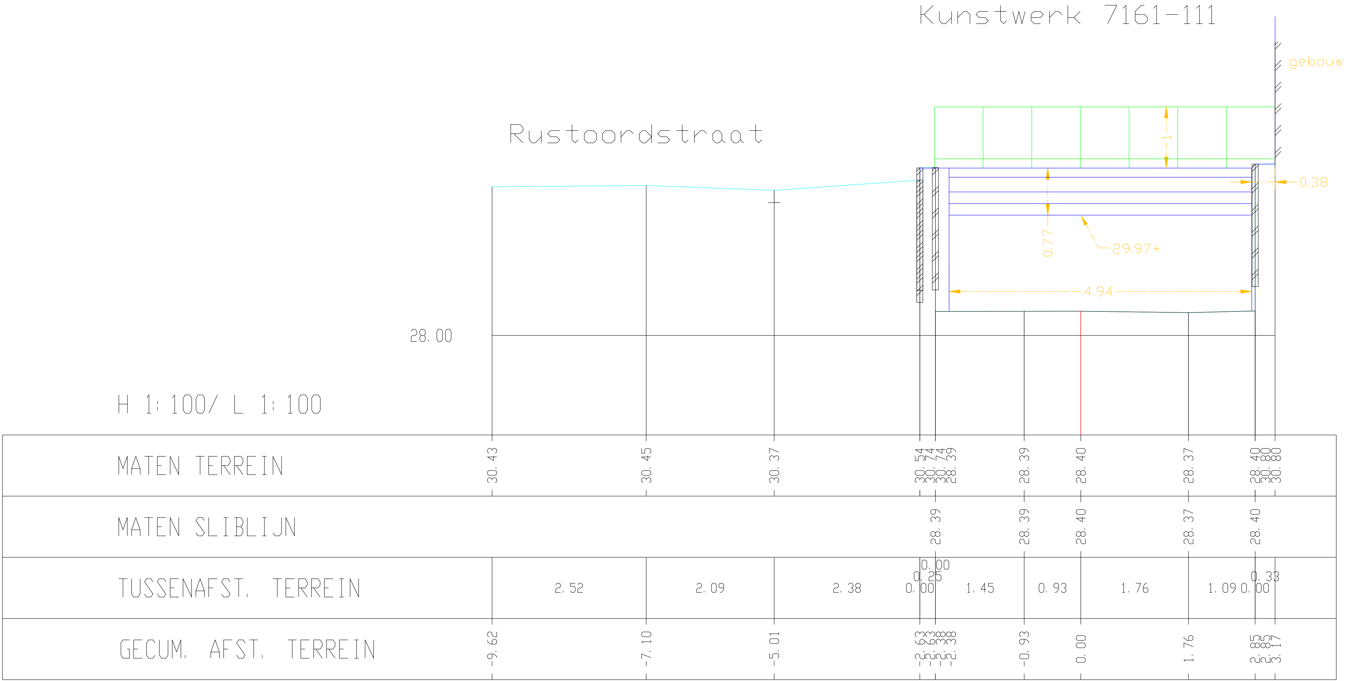
Kleine Gete, Dwarsprofiel 110
