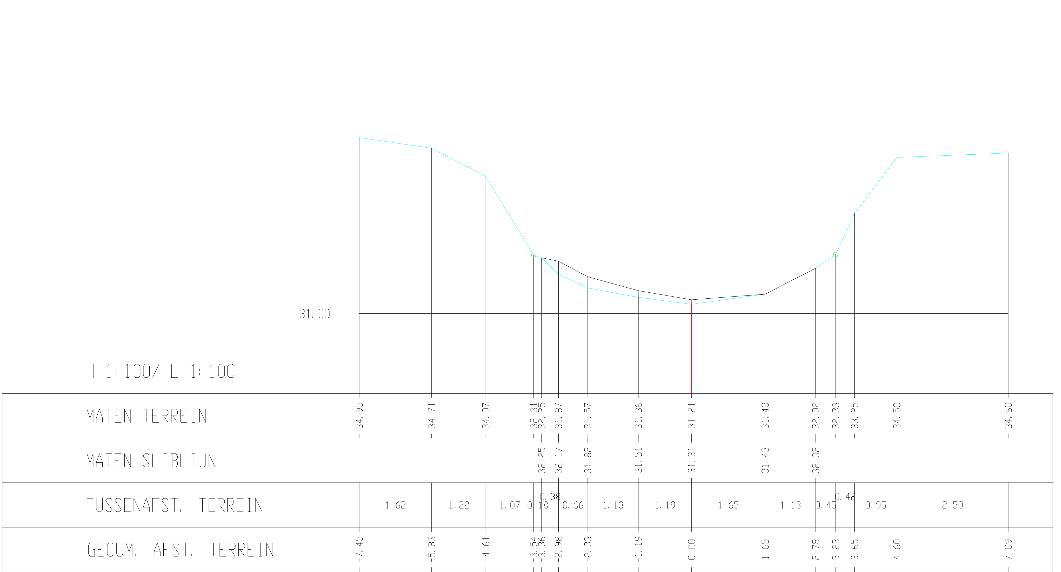
Kleine Gete, Dwarsprofiel 214
