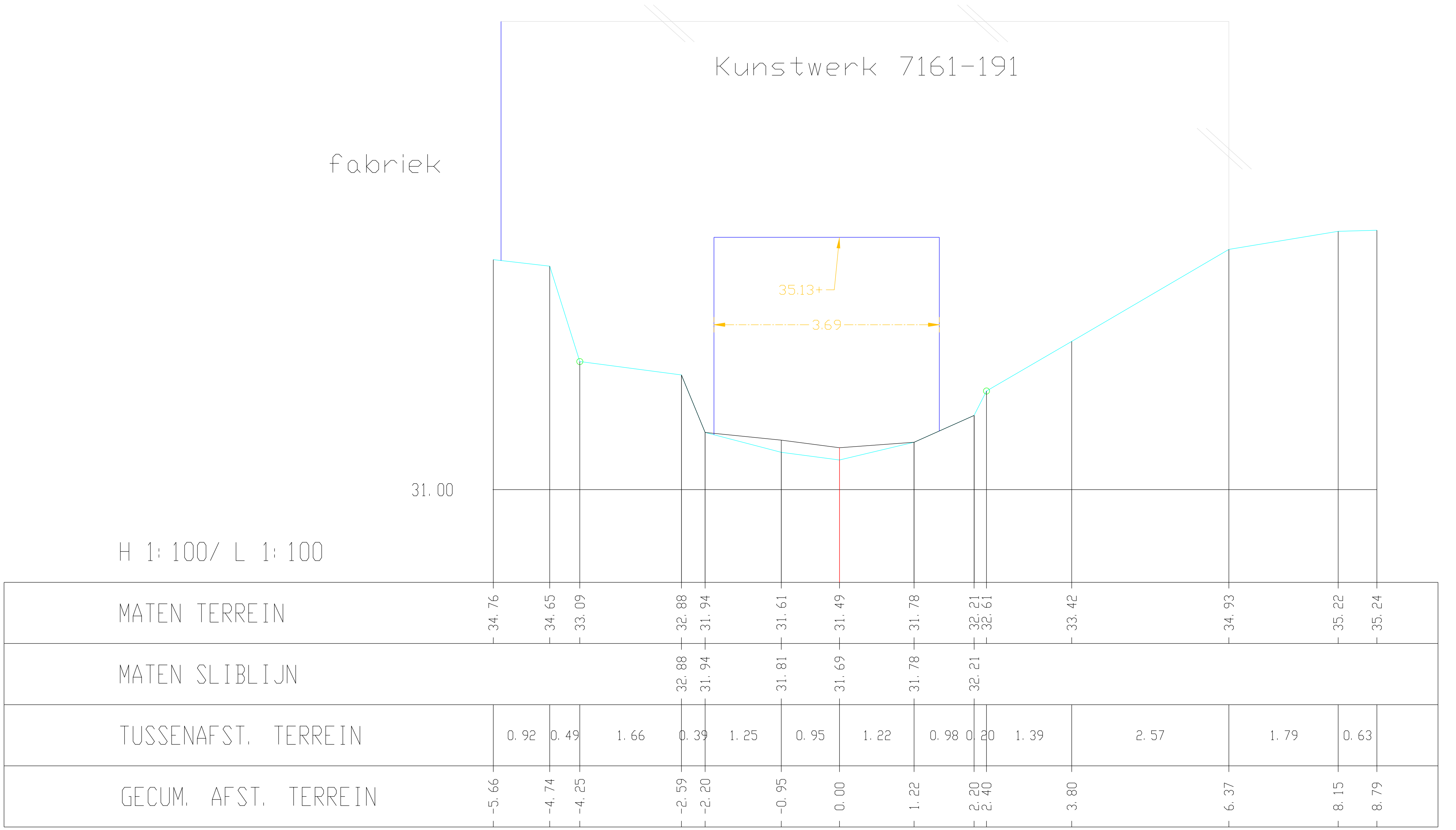
Kleine Gete, Dwarsprofiel 224
