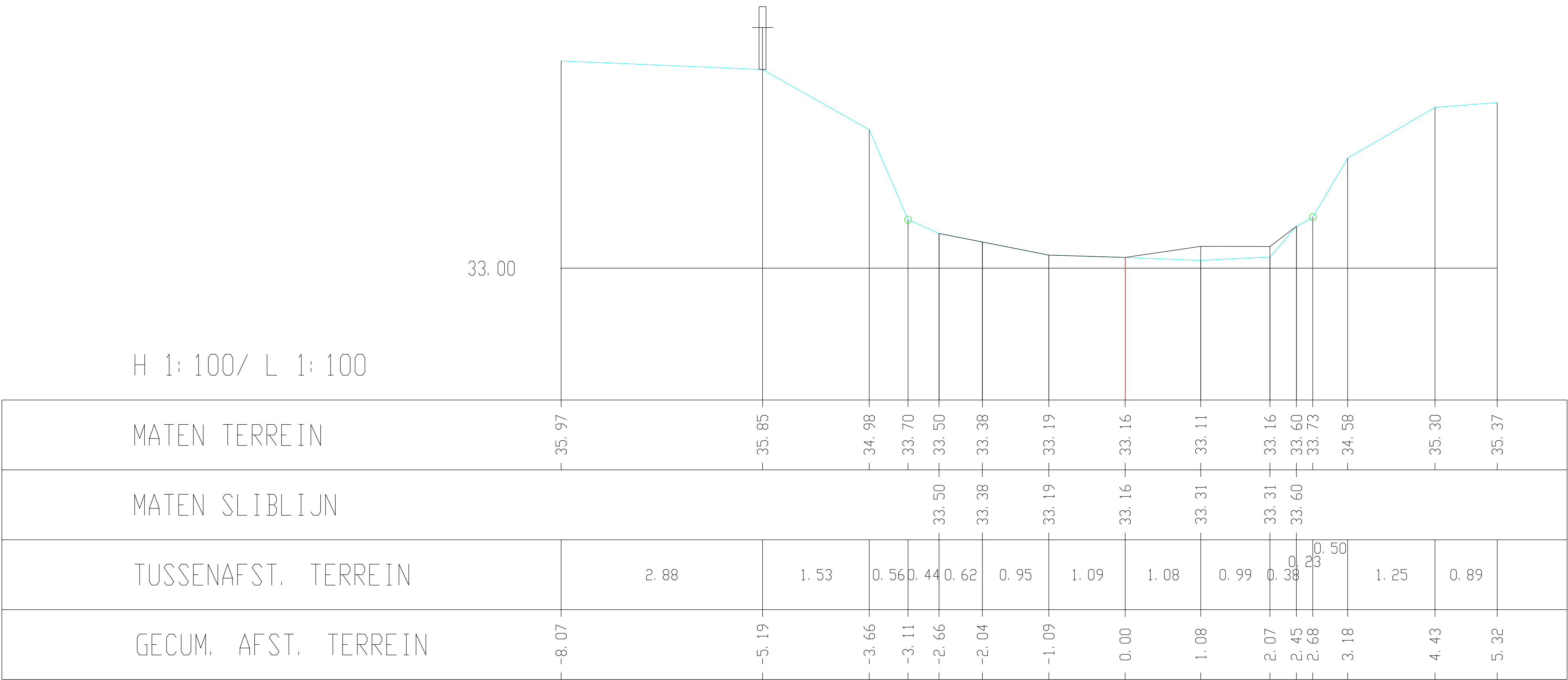
Kleine Gete, Dwarsprofiel 230
