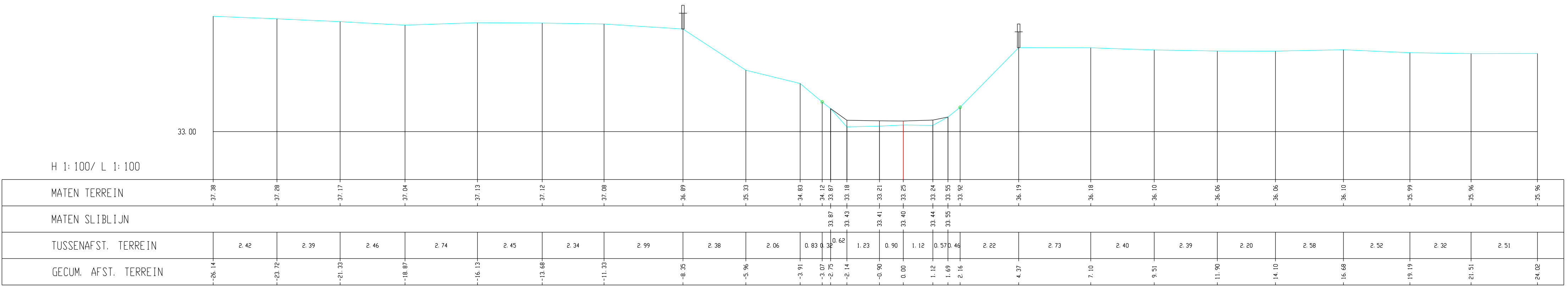
Kleine Gete, Dwarsprofiel 243
