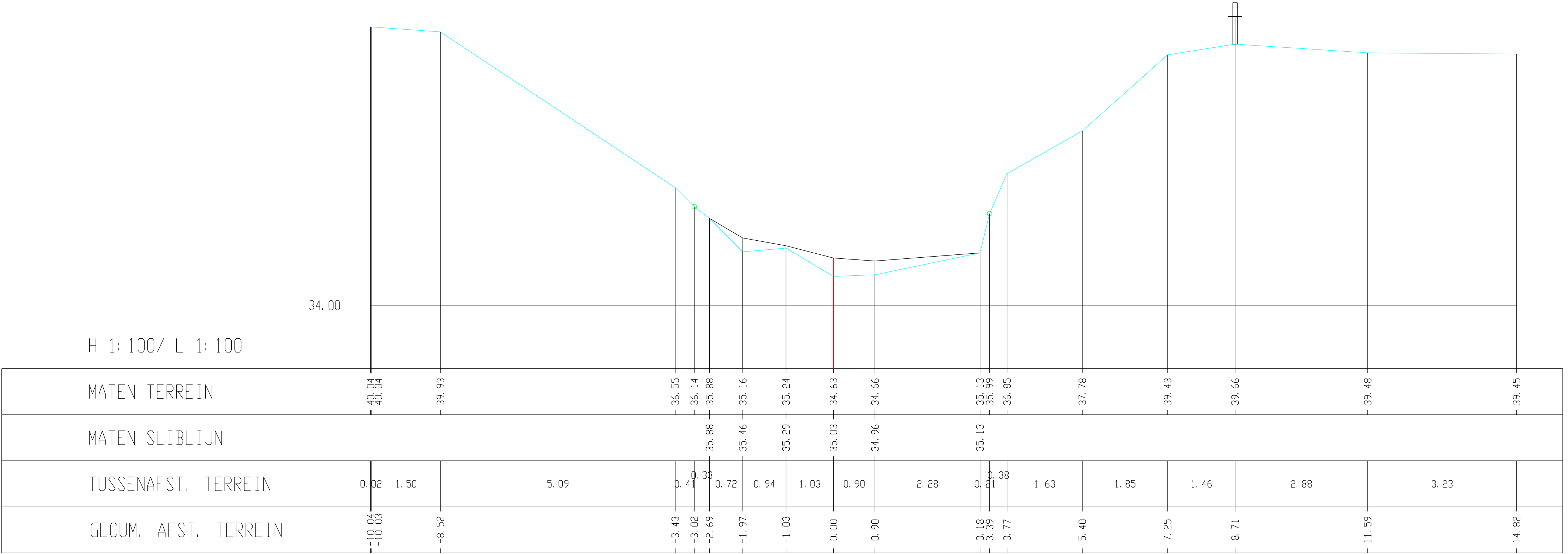
Kleine Gete, Dwarsprofiel 287
