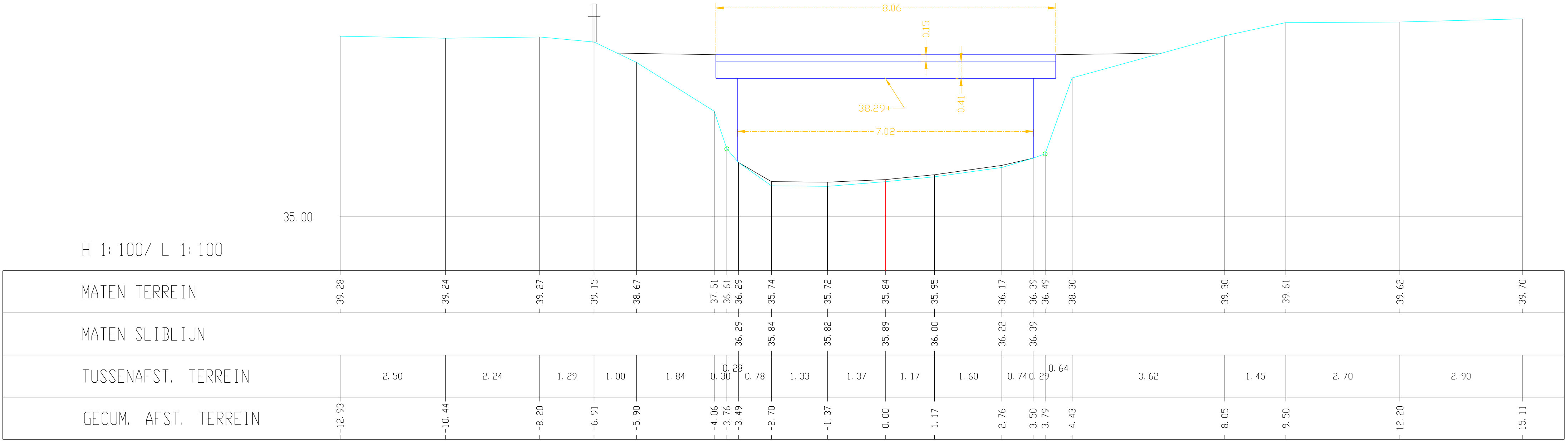
Kleine Gete, Dwarsprofiel 297
