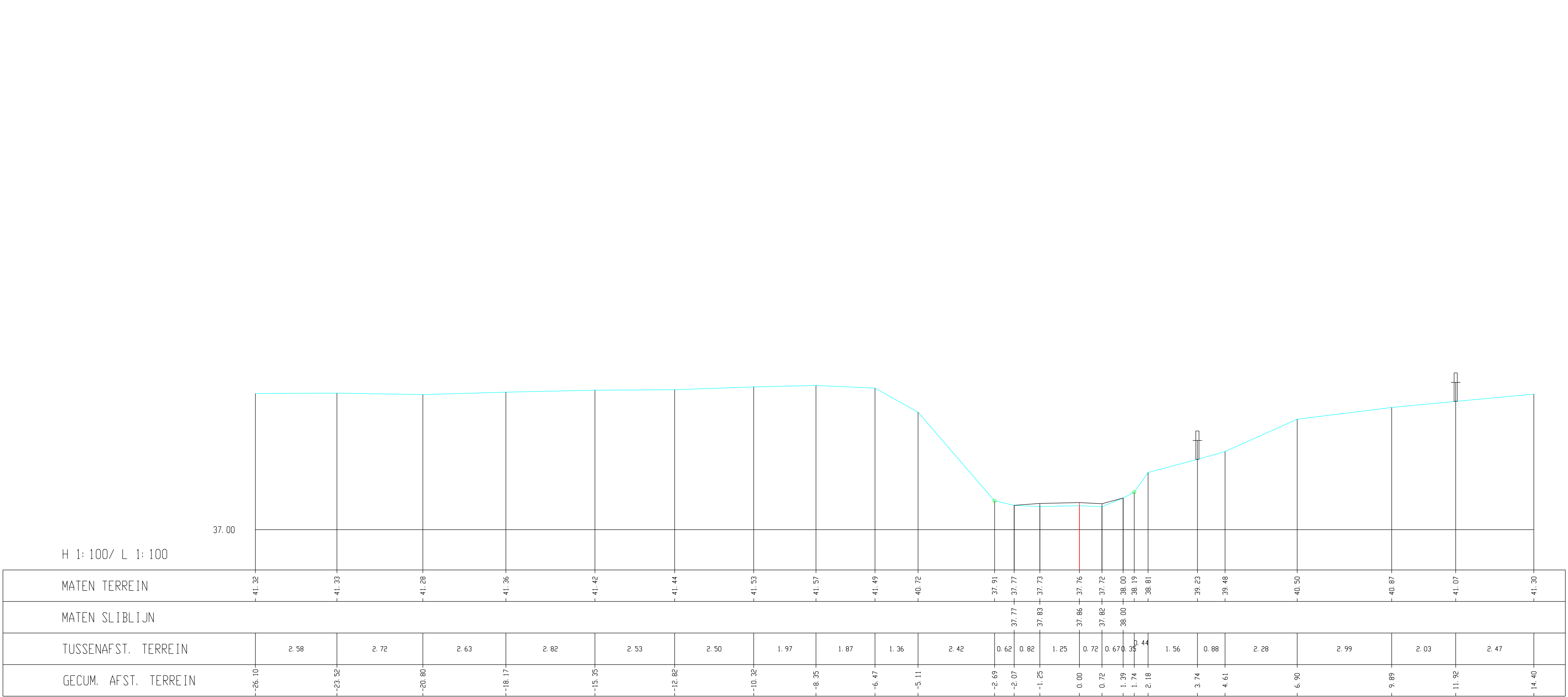
Kleine Gete, Dwarsprofiel 323
