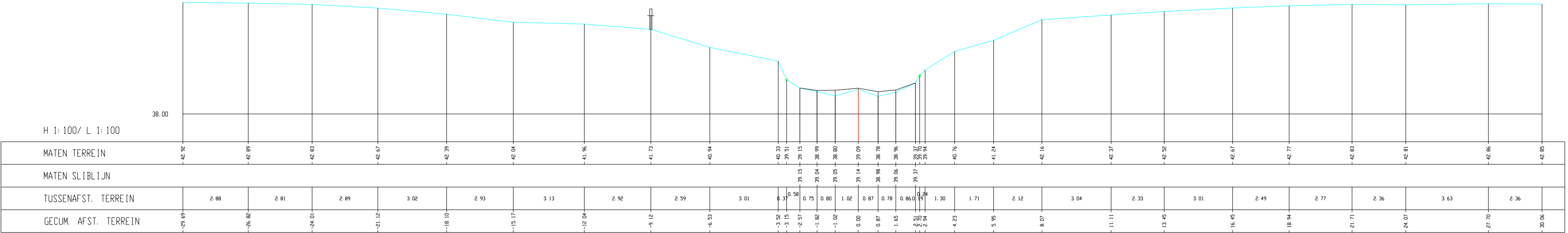
Kleine Gete, Dwarsprofiel 341
