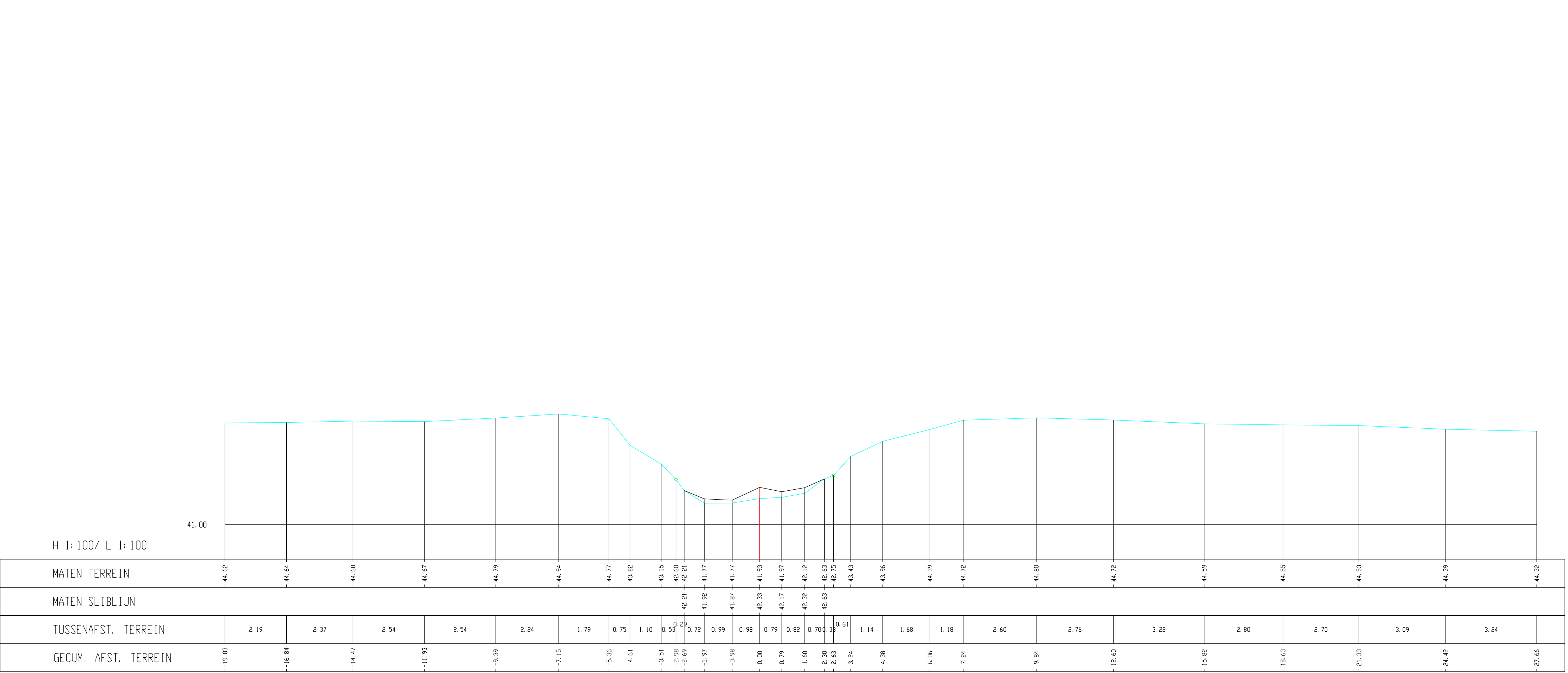
Kleine Gete, Dwarsprofiel 360
