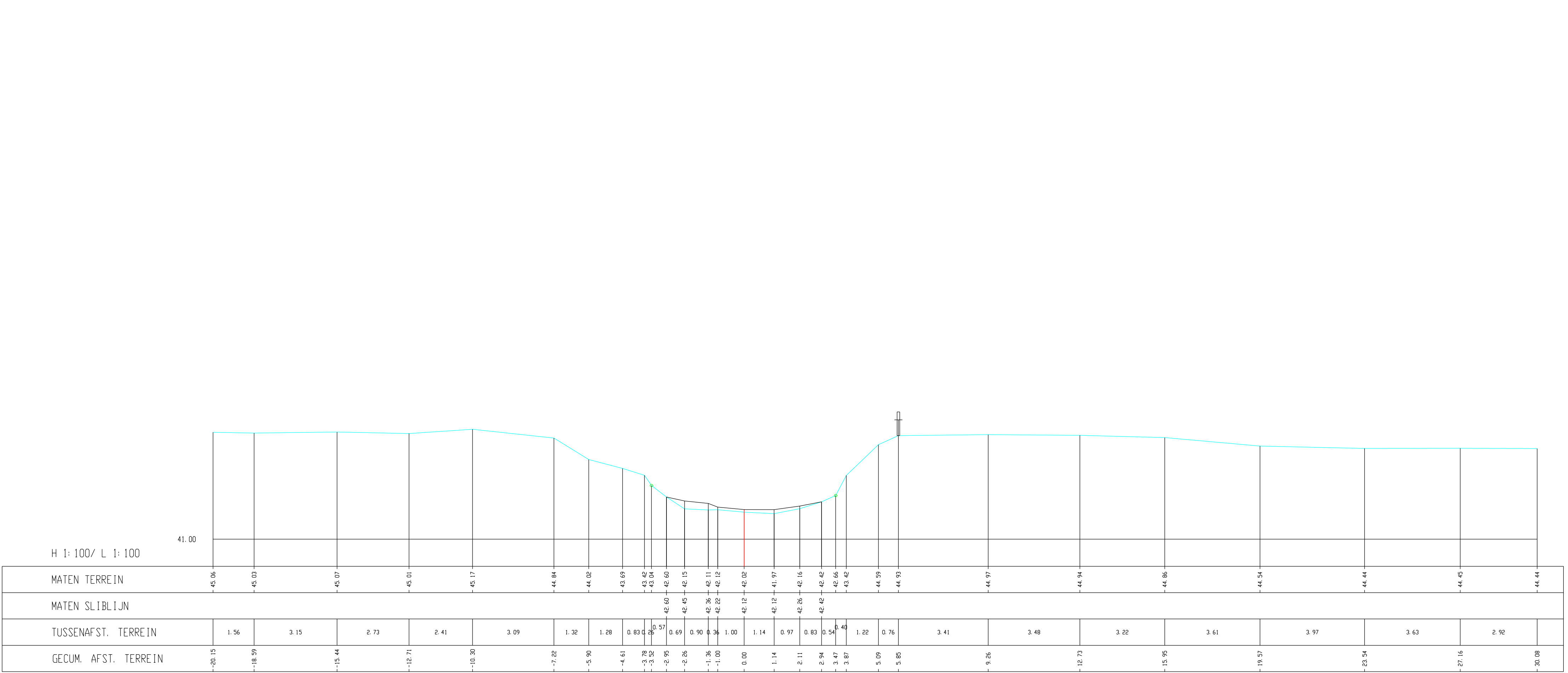
Kleine Gete, Dwarsprofiel 361
