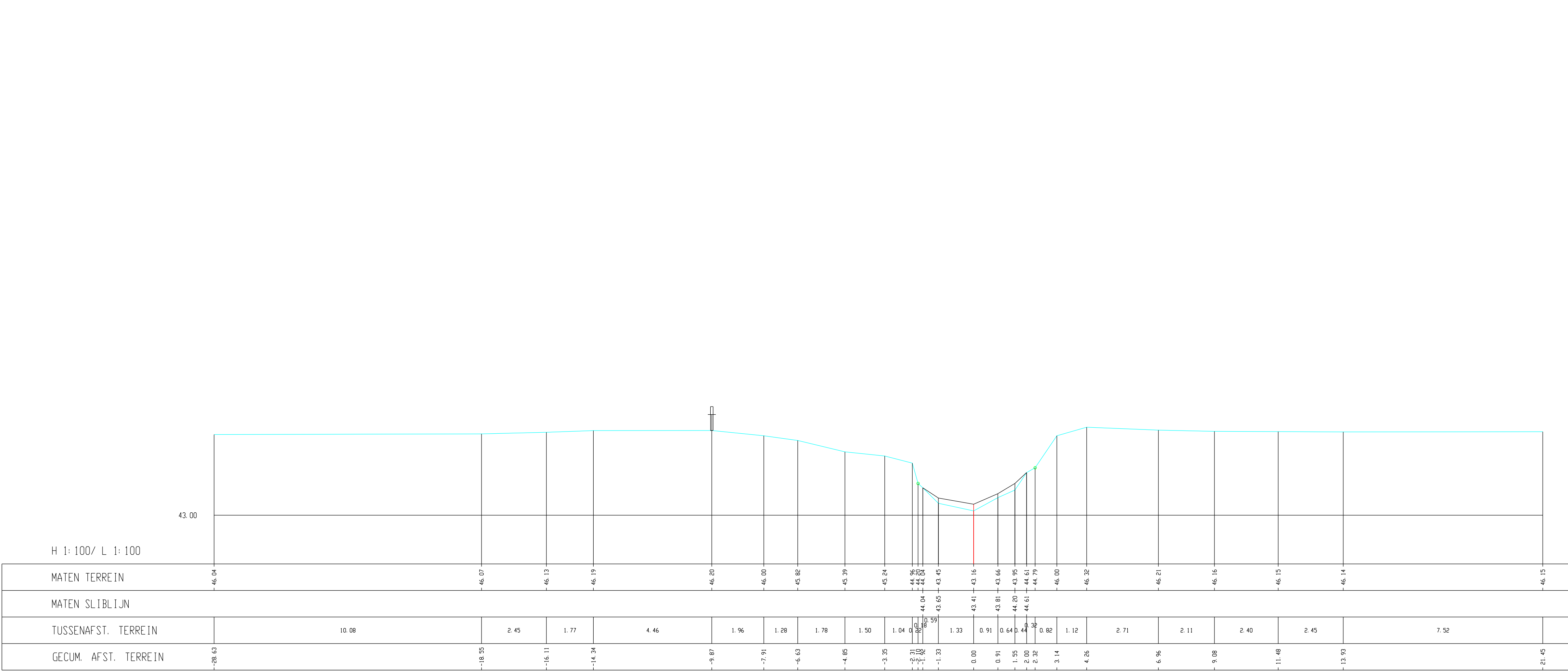
Kleine Gete, Dwarsprofiel 394
