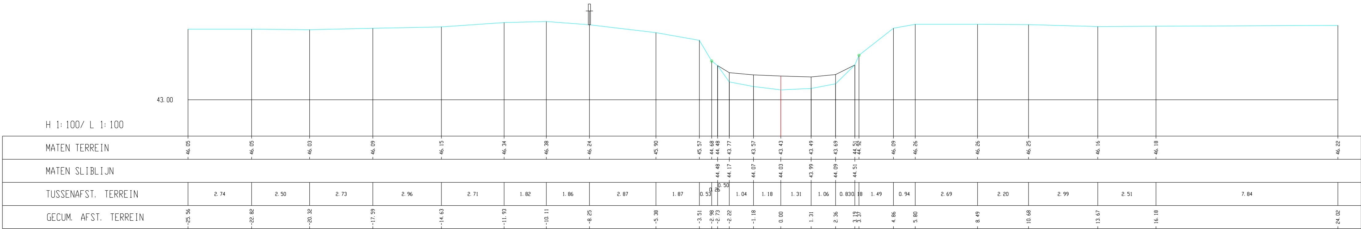
Kleine Gete, Dwarsprofiel 395
