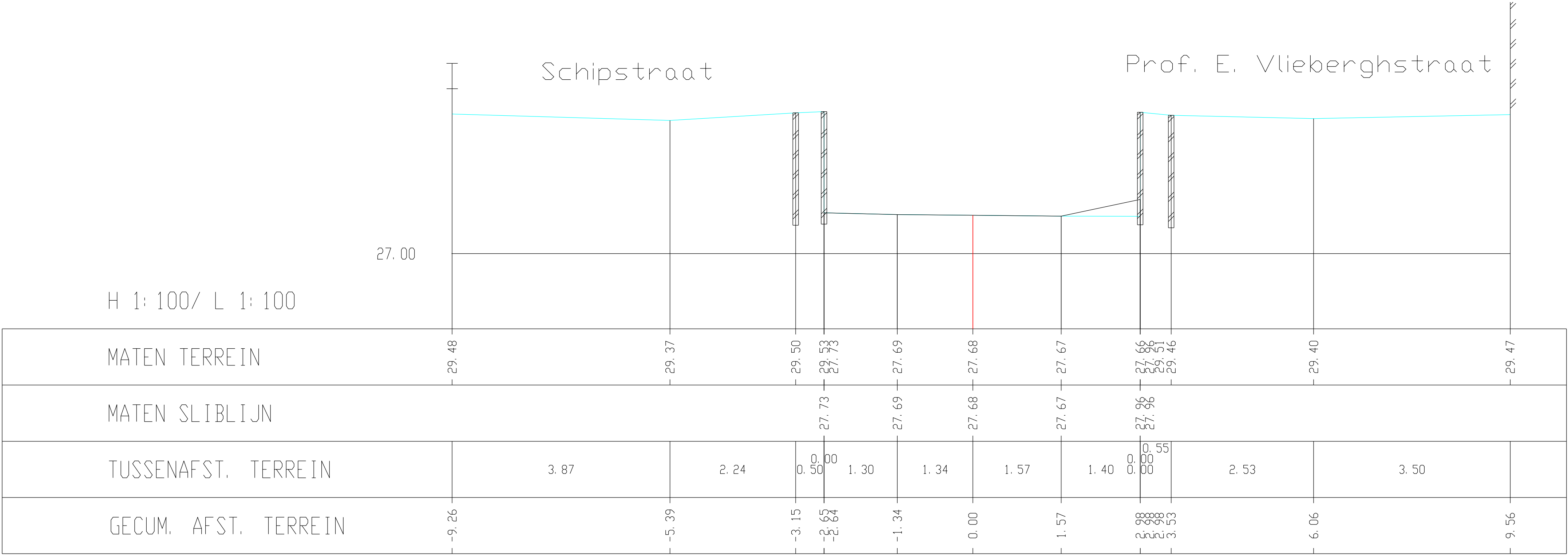
Kleine Gete, Dwarsprofiel 095
